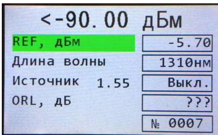
Рис. 22 Режим тестера. «Ручной»
