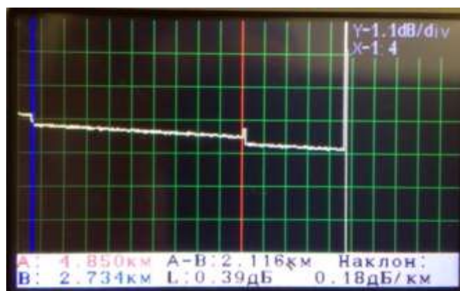
Рис. 14 Измерение длины и затухания участка линии
