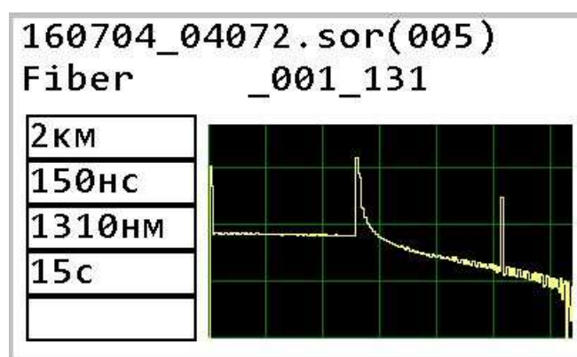
Рис. 20 Сохранённая рефлектограмма
