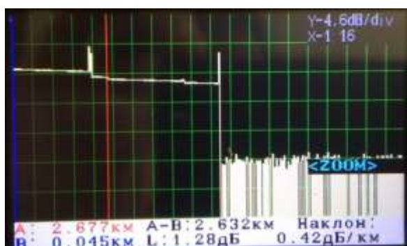
Рис. 13 Изменение масштаба рефлектограммы.
