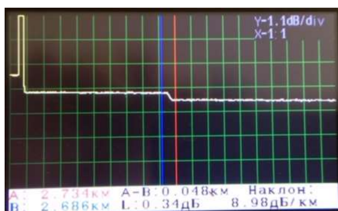
Рис. 15 Измерение затухания на неоднородности
