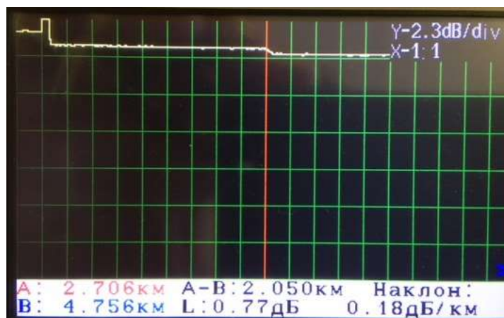
Рис. 18. Просмотр события 2 на графике рефлектограммы
