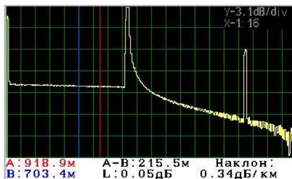
Рис. 12 Просмотр рефлектограммы.
