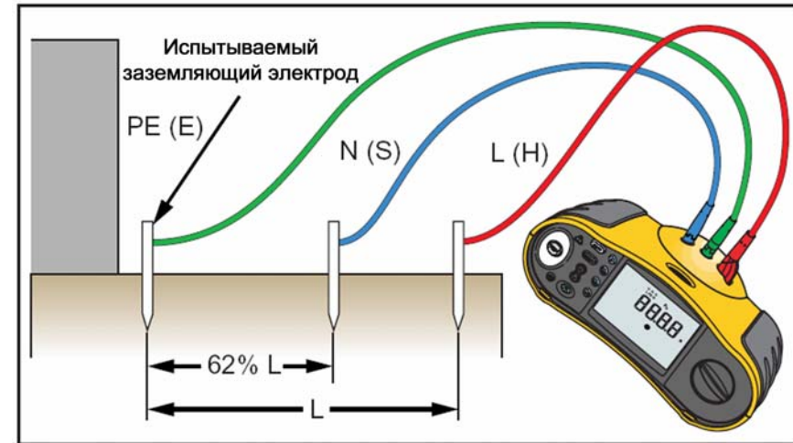
Рисунок 17. Подключение при измерении сопротивления заземления
