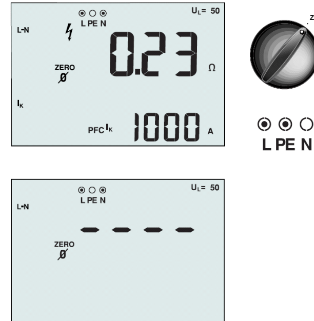
Рисунок 10. Дисплей при измерении сопротивления контура/провода и при установке нуля/Положение переключателя и клемм
