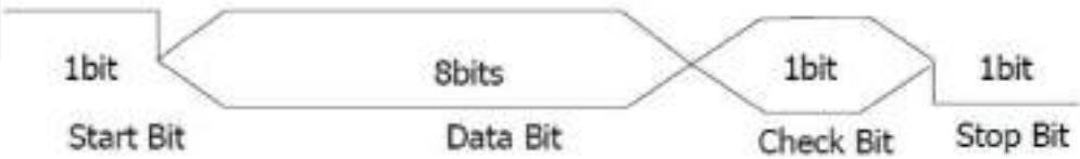
Триггер UART
