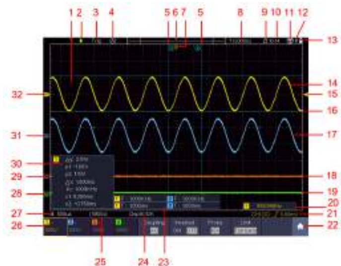
Рисунок 3-5 Интерфейс дисплея
