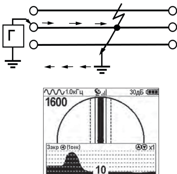
Рис.А.3 КЗ-одноф зное
